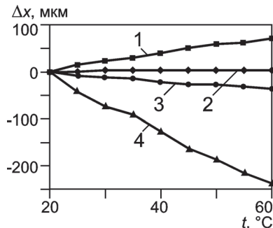
Рис. 3. Дополнительная температурная погрешность нуля струнных датчиков в следующих режимах работы:
